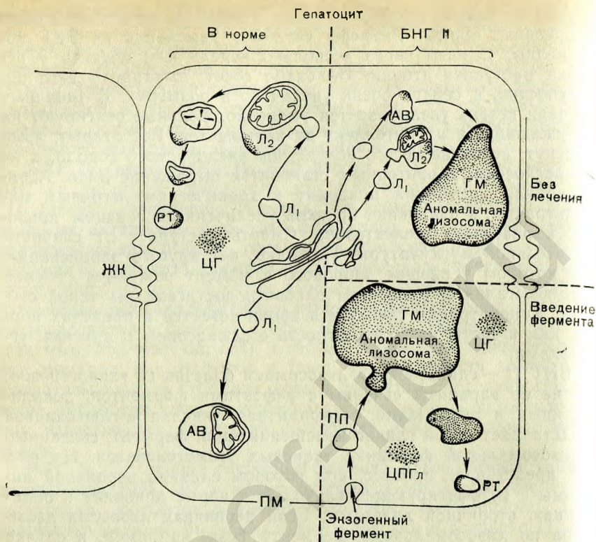
Рис. 7-18. Лизосомальный механизм.
